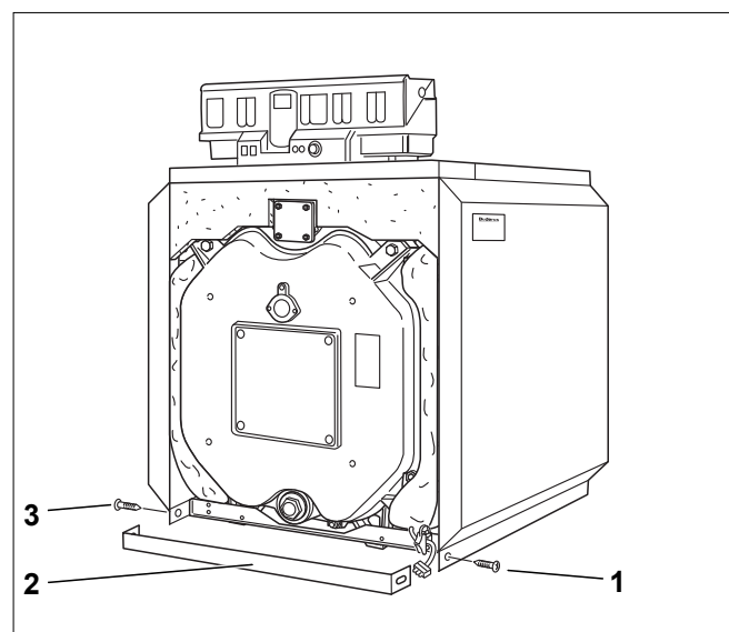
Рис. 38 Монтаж передней цокольной планки
