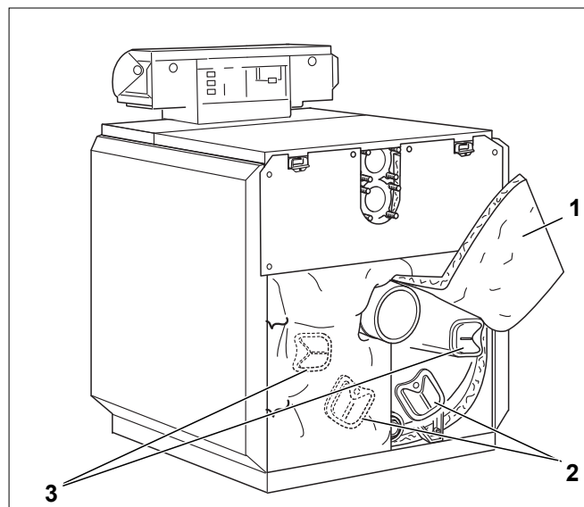
Рис. 52 Демонтаж крышек люка для чистки
