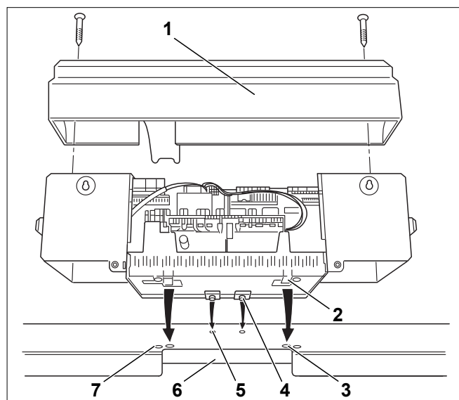
Рис. 43 Монтаж системы управления
