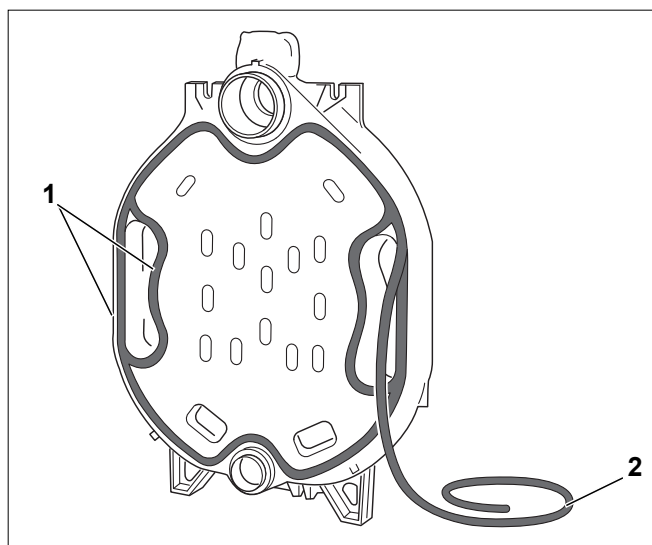
Рис. 11 Укладка уплотнительного шнура (шнур КМ)
