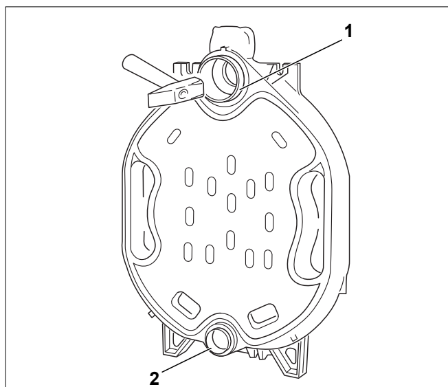
Рис. 9 Установка ниппеля
