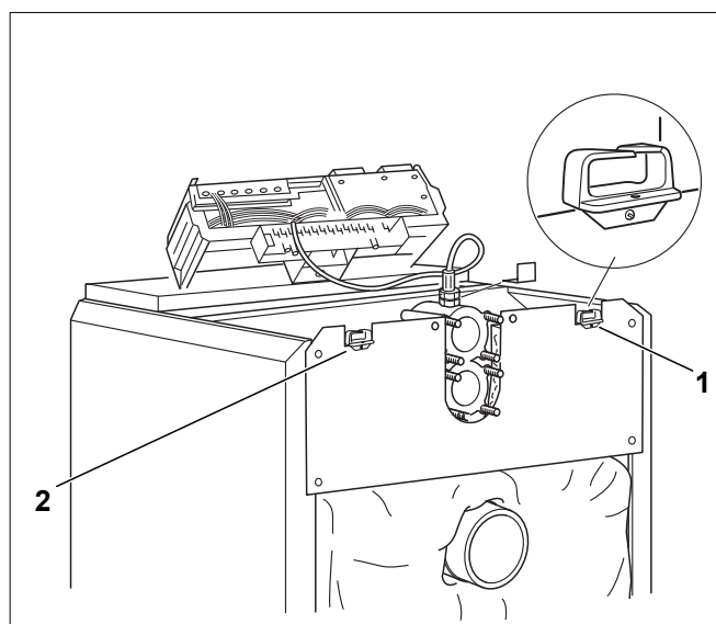
Рис. 46 Электрическое подключение
