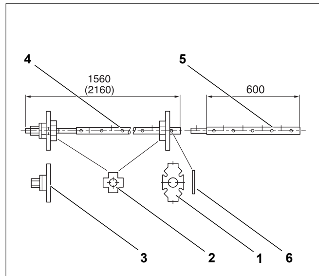
Рис. 1 Стяжной инструмент, размер 2.2
