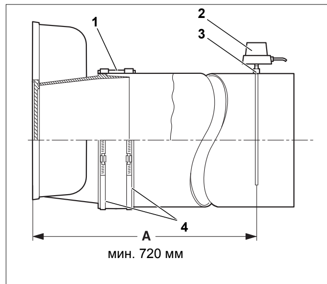
Рис. 29 Подсоединение к дымовой трубе
