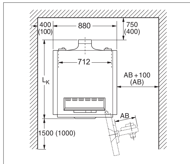
Рис. 4 Помещение с котлом
